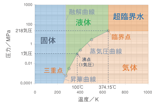
図1: 水の状態図
